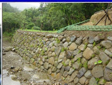
砌石護岸
