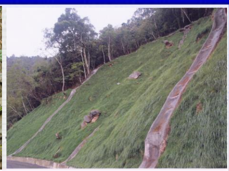
掛網噴植
