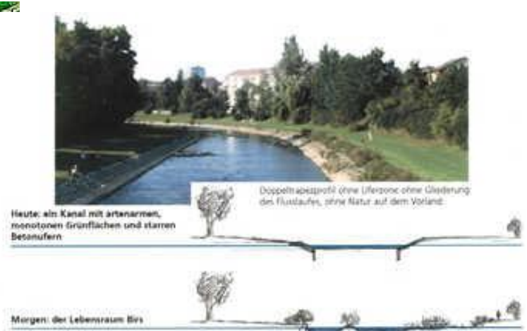
Reich gegliedertes Flussbett mit tiefen Becken, Flachwasserzonen und vielfältigen wechsellagernden Ständen; Ufer und Wasser sind vernetzt
